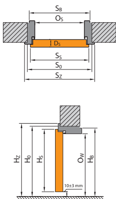
■ OŚCIEŻNICA STALOWA
